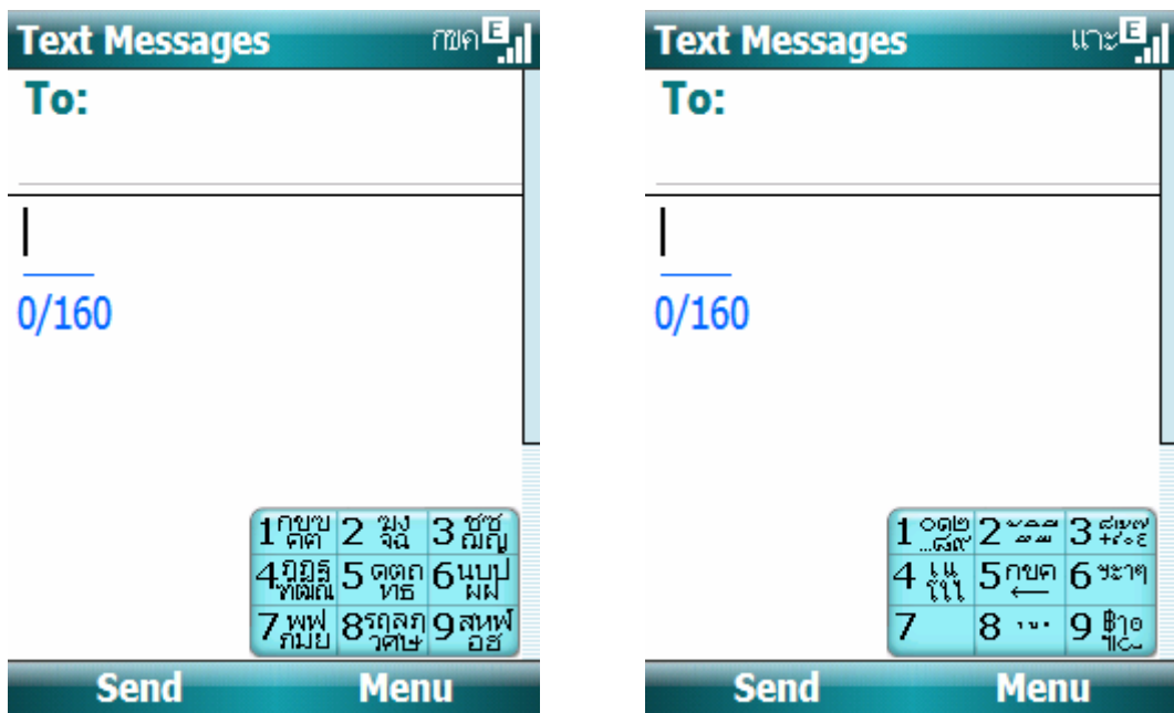
รูป Keyboard help ขณะพิมพ์วนจากปุ่มตัวเลข
